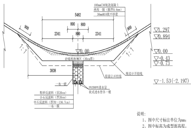
图1 总干渠排水改造变更后断面图
