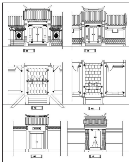
图1 多种中式屏门CAD效果图
