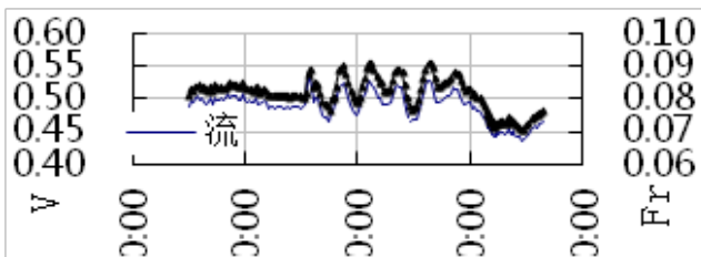
图1 北拒马河2015~2016年冰期输水期间闸前水流流速和水流弗汝德数变化曲线
