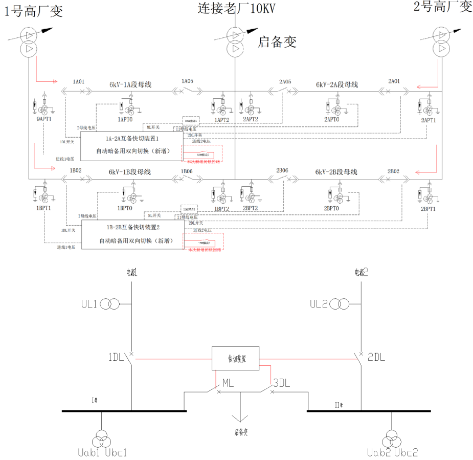
注：新增两台快切装置工作原理接线图所示，正常运行时：1DL 合位，进线1 通过 1DL 向 I 母供电；2DL 合位，进线2 通过 2DL 向 II 母供电；ML 分位，3DL 可以在分位也可以在合位，控制通过压板实现，I 母、II 母通过 ML 形成互为备用。当 3DL 分位，3DL 跟随 ML 逻辑分合，当 3DL 合位，则断开压板，3DL 跟随 ML 动作逻辑不变，但是实际分合都通过断开压板不予以动作
