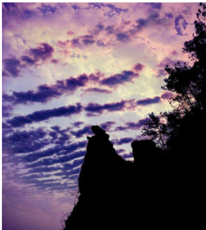
图1 天鸡晓月
