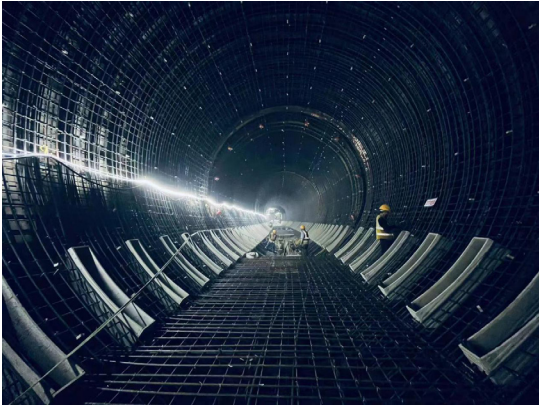
图 3-2 钢筋安装
