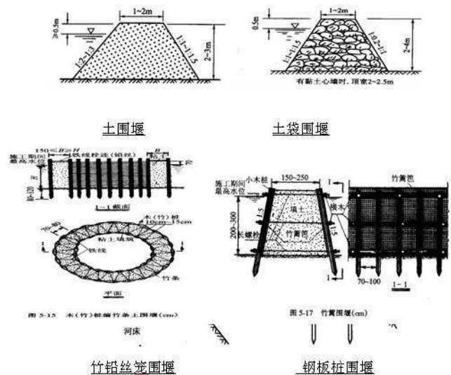
图1 不同类型的围堰施工技术
