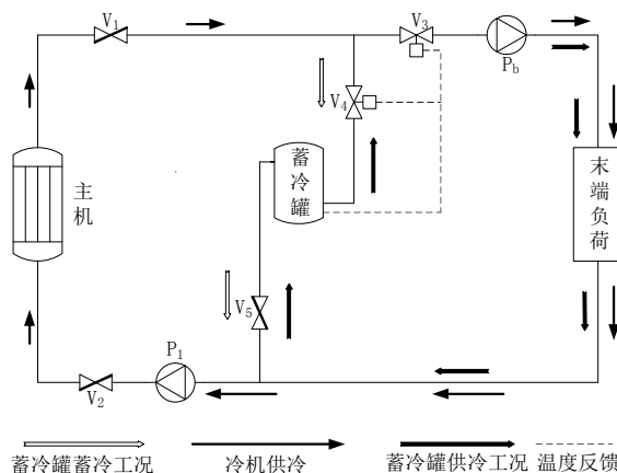
图 4 二级泵并联开式罐方案示意图
