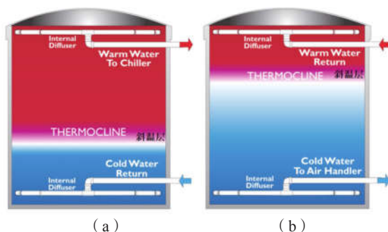
图 1 单冷罐水蓄冷系统示意图
