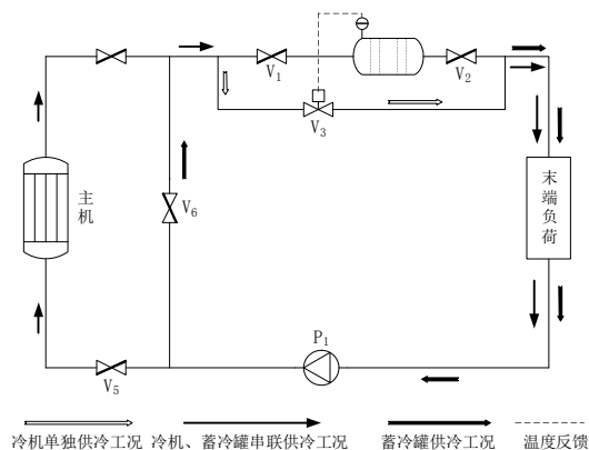
图 3 一次泵串联闭式罐方案示意图
