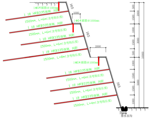
图1 边坡支护图示
